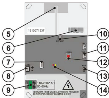
Abb. 3: 5 – Antenne; 6 – Seriennummer; 7 – miniUSB-Anschluss; 8 – Anschluss für Backup-Batterie; 9 – Klemme für Netzanschluss und Schutzfolie; 10 – Anschluss für externe Antenne; 11 – Anschlüsse für Sabotagekontakt; 12 – LEARN-Taste; 13 – Klemme MAN für manuellen Start von Backup-Batterie; 14 – LED-Anzeigen
