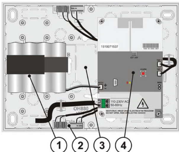
Abb. 2: 1 – Backup-Batterie; 2 – Sabotagekontakte; 3 – unterer Teil der JA-194PL-Box; 4 – JA-150R-Modul
